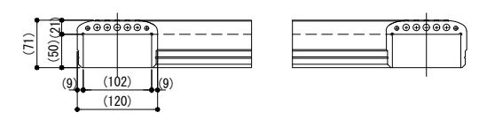
砂場受(コーナー) S=1/5
