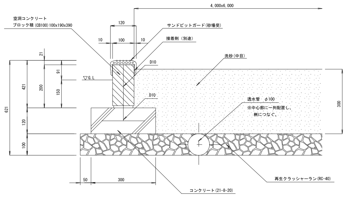
断面図 S=1/5
