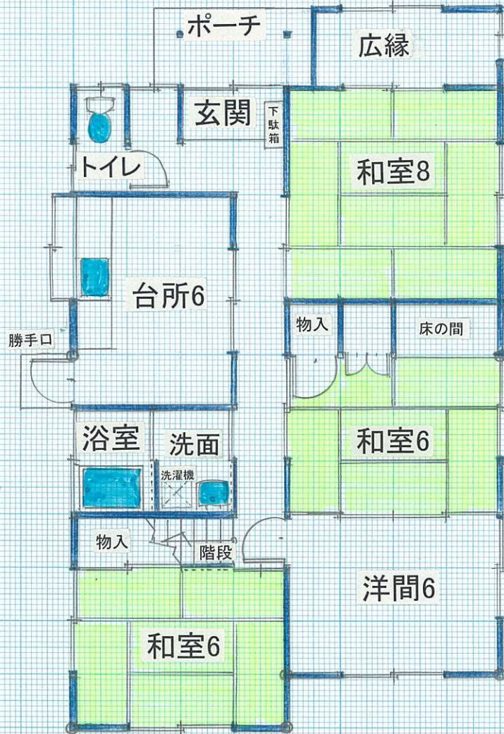
1階平面図
