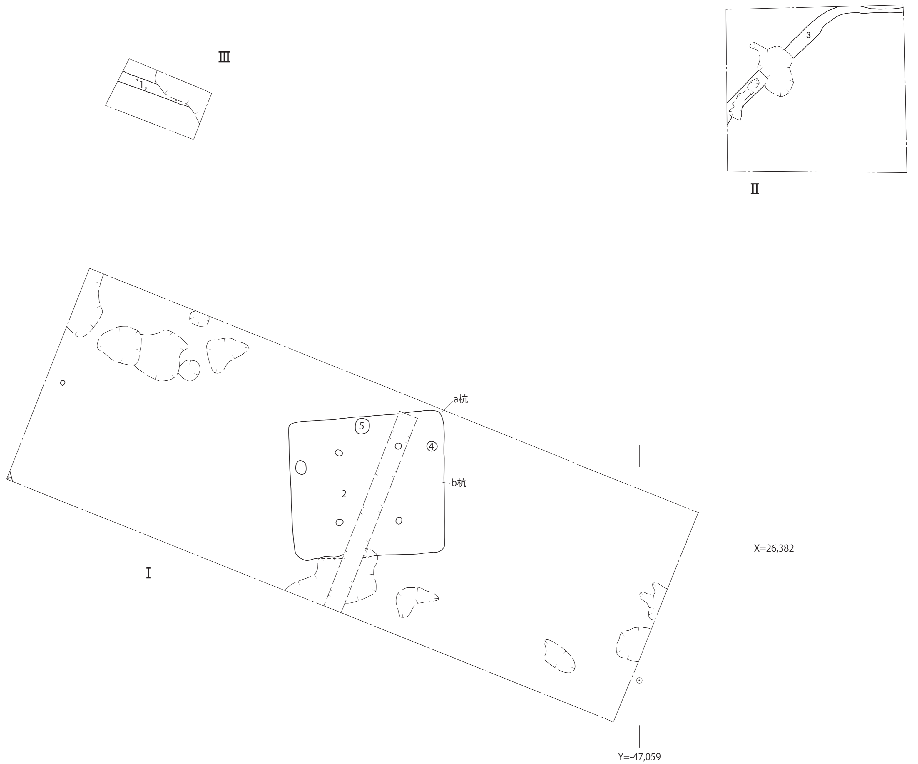
蔵数西野屋敷遺跡 第2次調査 略測図(1/100)
