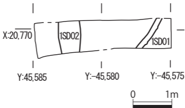
志藪ノ内遺跡 第1次調査 略測図 (1/100)
