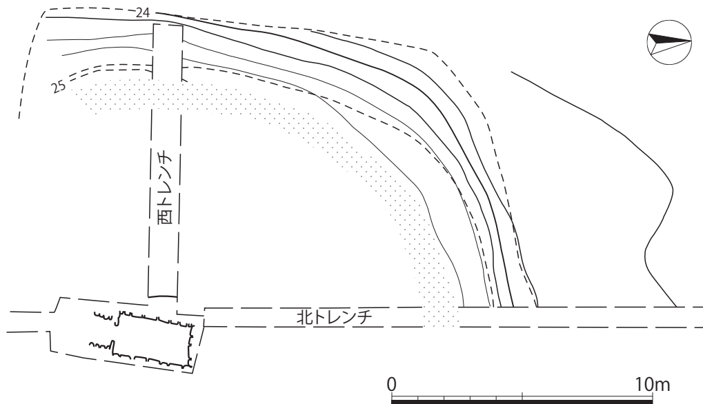
瑞王寺古墳 略測図(1 / 200)
