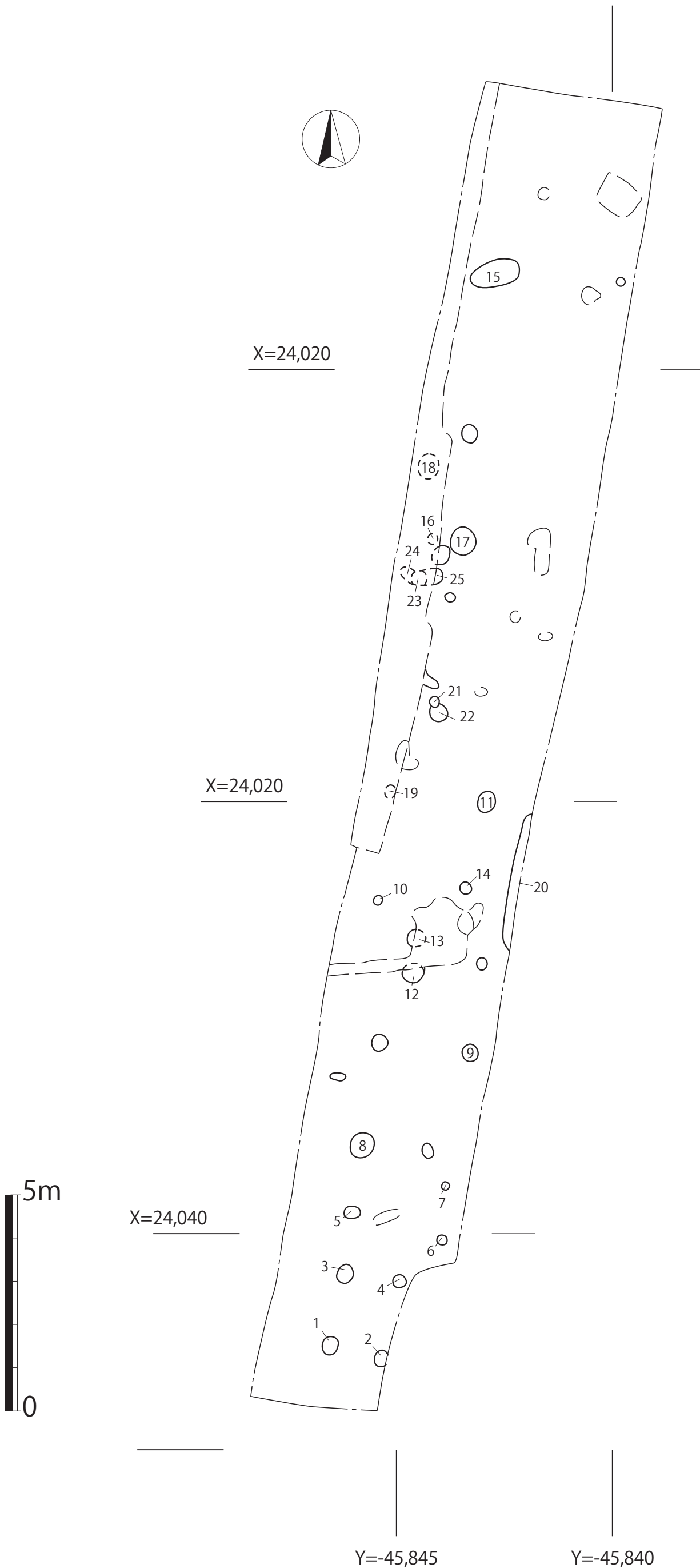
羽犬塚山ノ前遺跡第2次調査 遺構略測図(1 / 100)
