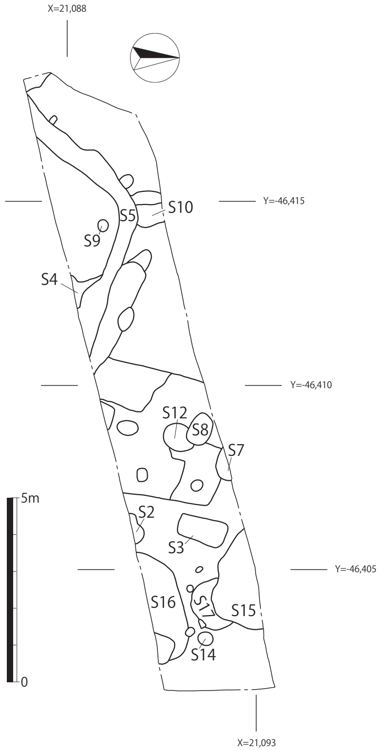
裏山遺跡第3次調査 遺構略側図(1 / 100)
