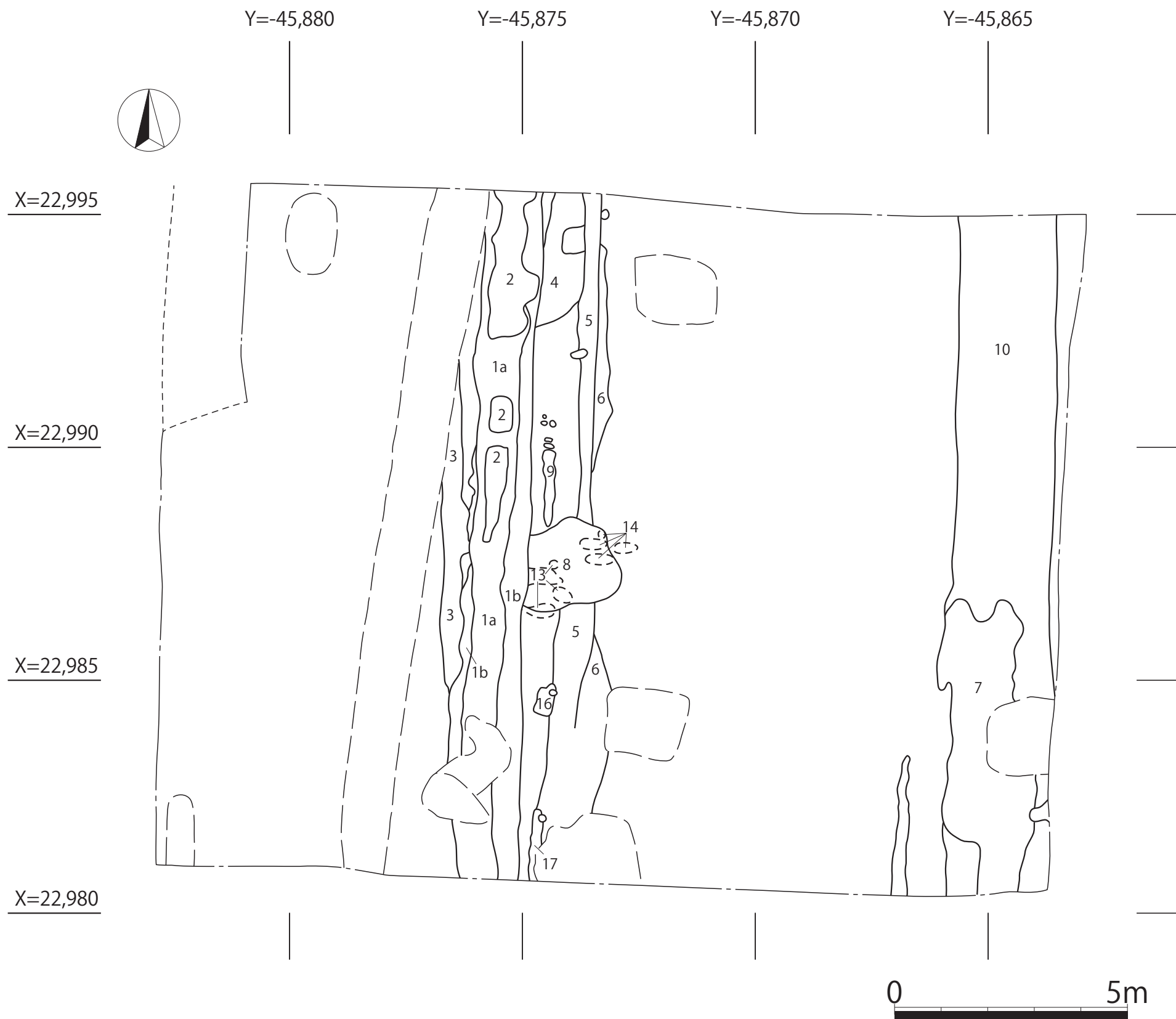
山ノ井南野遺跡第4次調査 遺構略測図(1 / 100)
